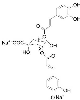
图1 异绿原酸A钠的结构式
