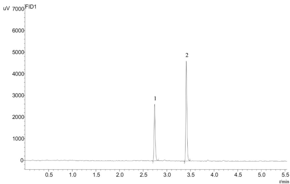
图B.1 甲醇和乙酸乙酯（10 \mu\text{g/mL} ）混合标准溶液的气相色谱图
